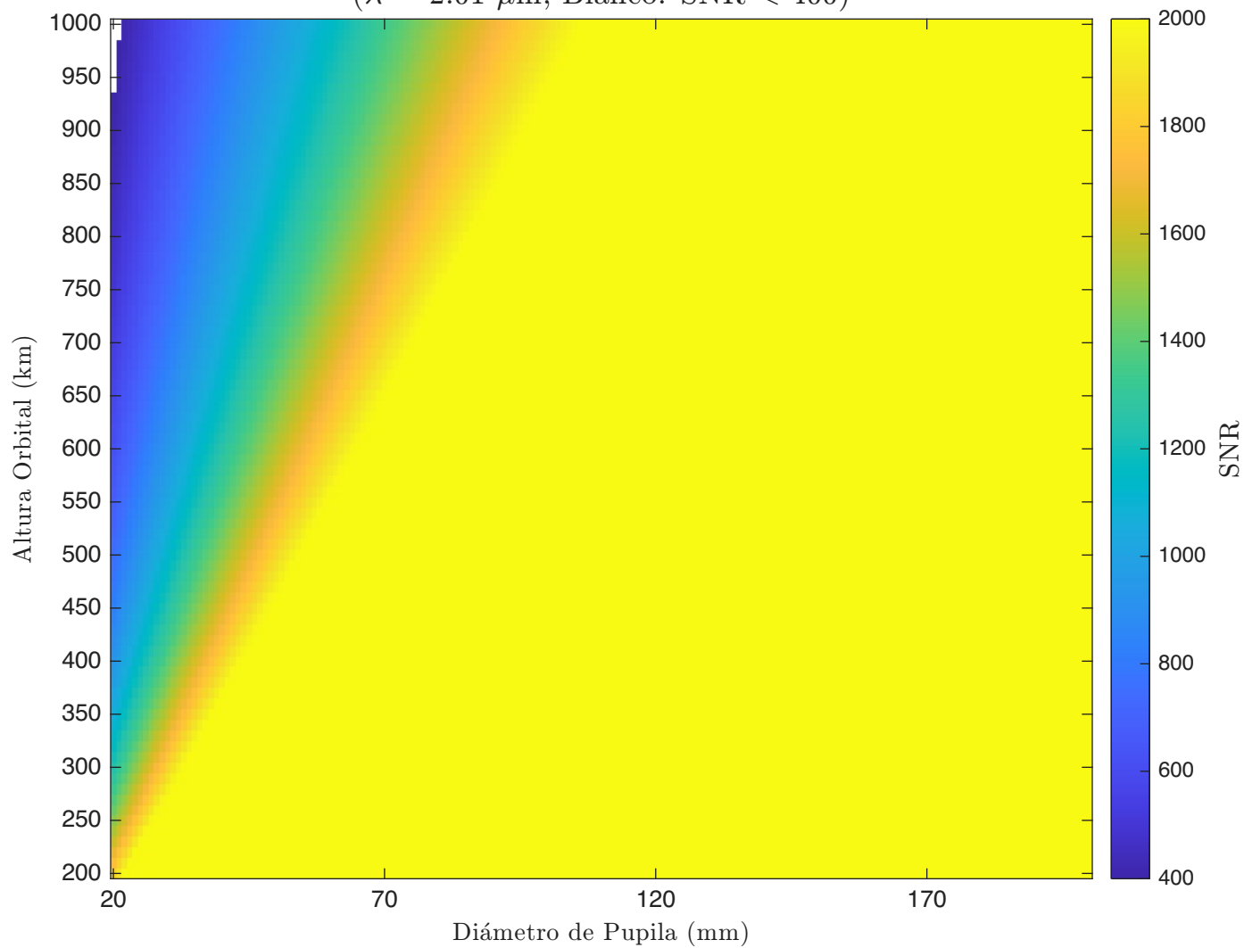
SNR - TMA - Detector 2 ( \lambda = 2.01 \mu\text{m} , Blanco: SNR < 400)
